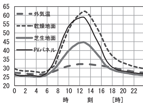
図3 各部表面温度 東京8月1日
